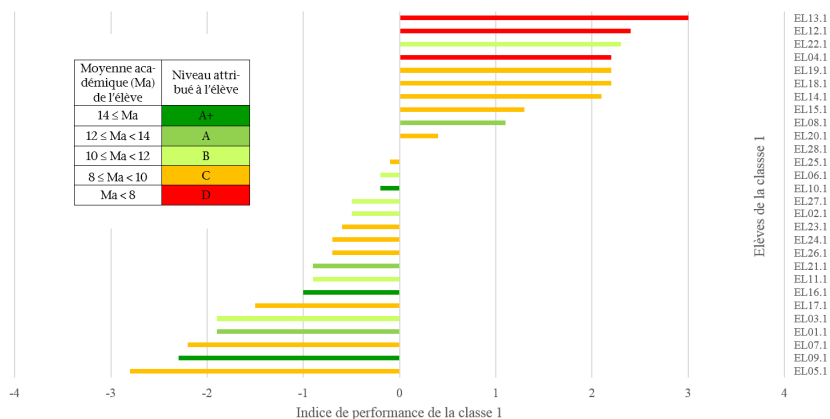
Figure 2a • Ventilation du niveau des élèves en fonction de l'indice de performance pour la classe 1
