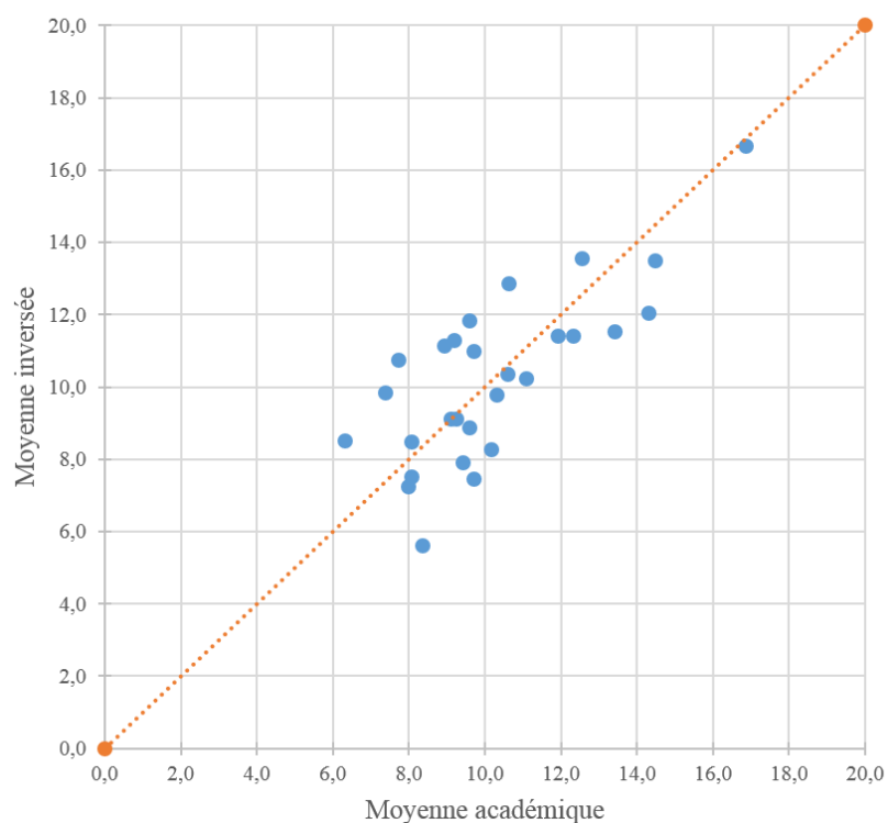
Figure 1a • Moyennes académiques (en abscisse) vs moyennes en classe inversée (en ordonnée) pour chaque élève de la classe 1
